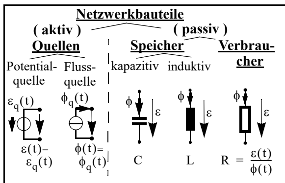
Abbildung 3. Übersicht der Netzwerkbauerelemente für die dynamische Modellbildung
